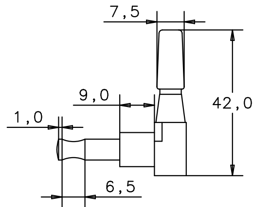
Seitenansicht von links side view left
