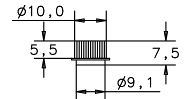
Vorderansicht / Rückansicht / Seitenansicht front view / back view / side view
