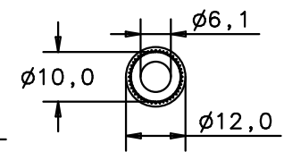
Untersicht bottom view
