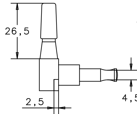
Seitenansicht von rechts side view right
